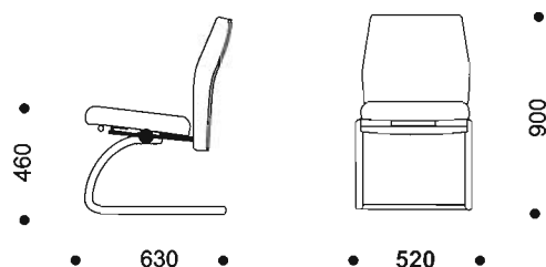
• GESS 10.050 FP S/B - Bajo, patín, sin brazos. • GESS 10.050 F S/B - Bajo, 4 patas, sin brazos. • (sistema oscilante)
