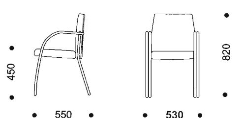
• GESS 9.050 F - Silla apilable, 4 patas, con brazos.
